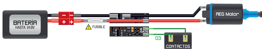
FIG 3. MONTAJE CON CAMBIO DE INSTALACIÓN (CABLEADO)
